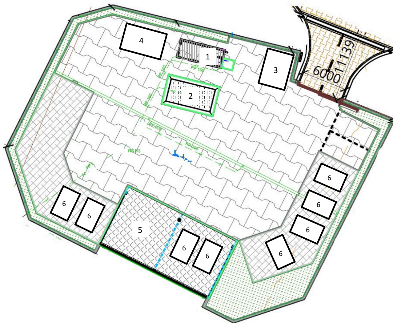
Příloha č. 1: Dispoziční řešení sběrného dvora
